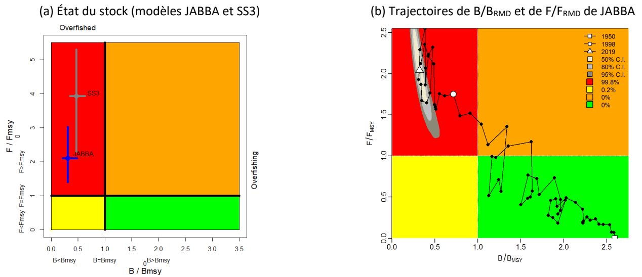
Figure 3. (a) Marlin rayé : État du stock de l’océan Indien issu des modèles d’évaluation JABBA (modèle bayésien de production excédentaire état-espace) et SS3 avec les intervalles de confiance (gauche) ; (b): Trajectoires (1950-2019) de B/B_{RMD} et F/F_{RMD} d’après le modèle JABBA. NB: SS3 se rapporte à SB/SB_{RMD} tandis que le résultat du modèle JABBA se rapporte à B/B_{RMD} .
